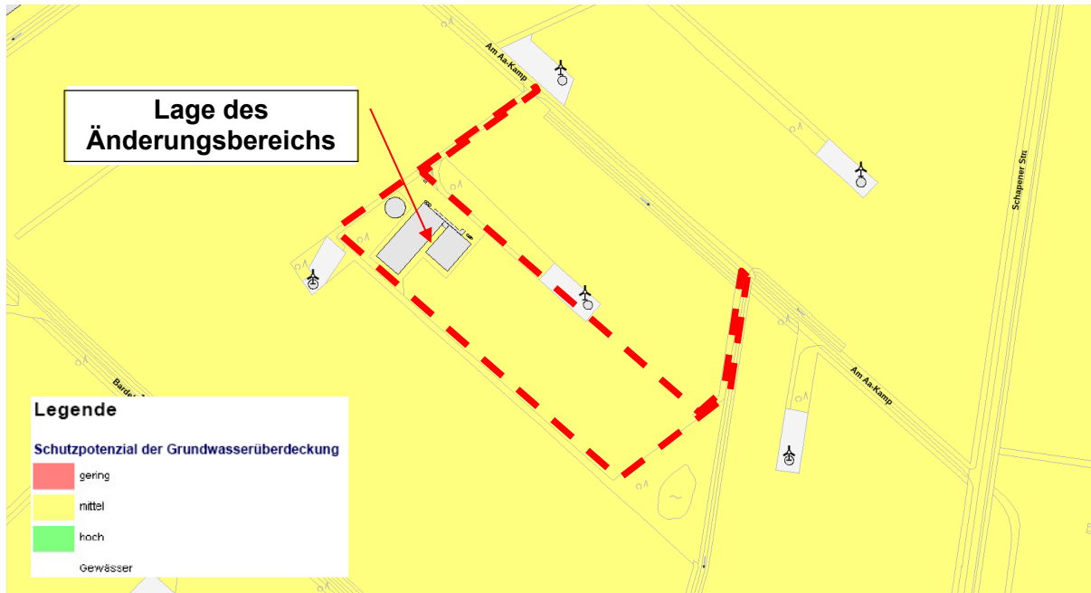
Abbildung 14: Schuttpotenzial der Grundwasserüberdeckung, unmaßstäblich (LBEG 2026)
