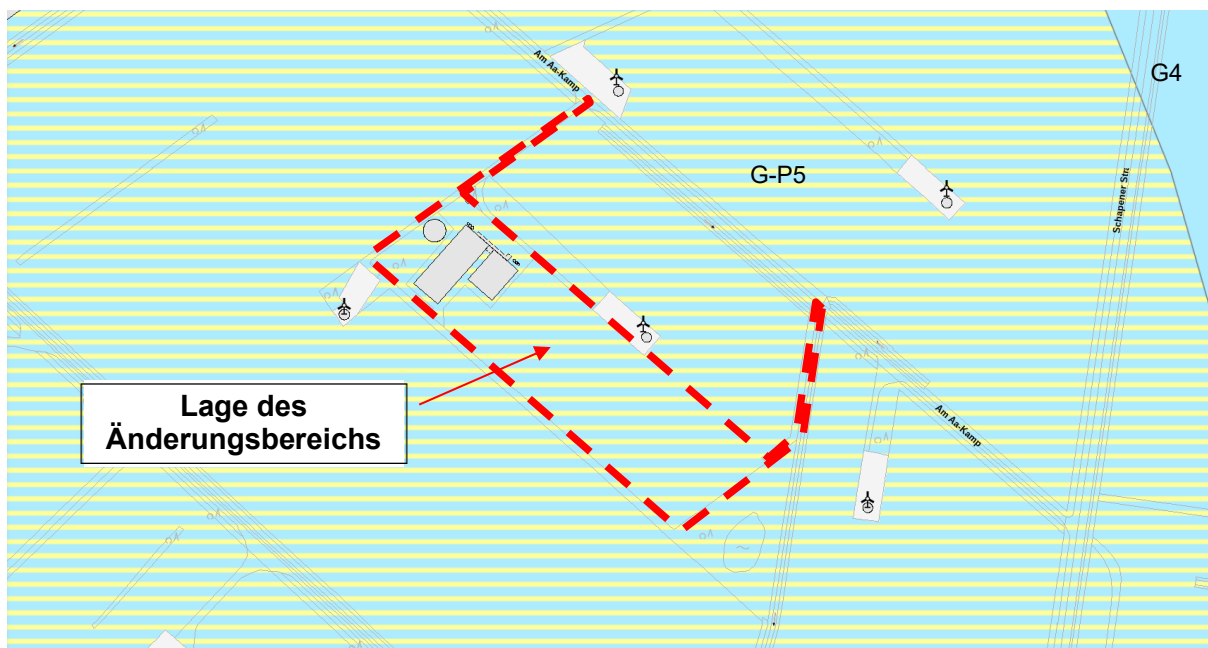
Abbildung 13: Schutzgut Boden - Bodenkarte, unmaßstäblich (LBEG 2026)
