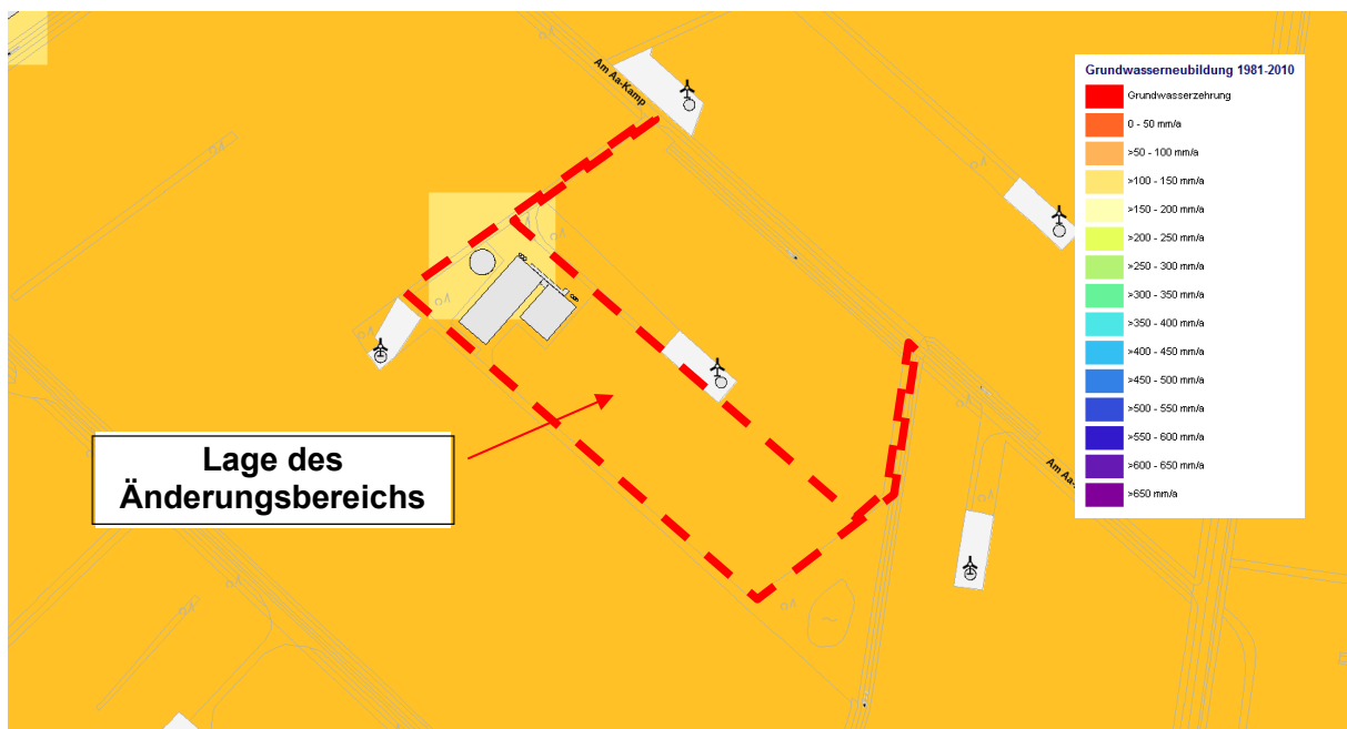
Abbildung 15: Grundwasserneubildung im Jahresmittel der Jahre 1991-2020, unmaßstäblich (LBEG 2026)
