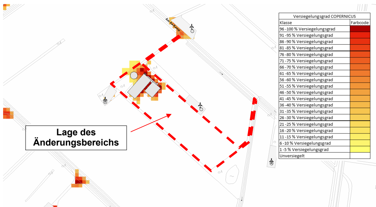
Abbildung 11: COPENICUS - Bodenversiegelung 2018; in %, unmaßstäblich (LBEG 2026)
