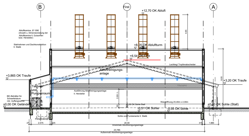
Schnitt B-B
