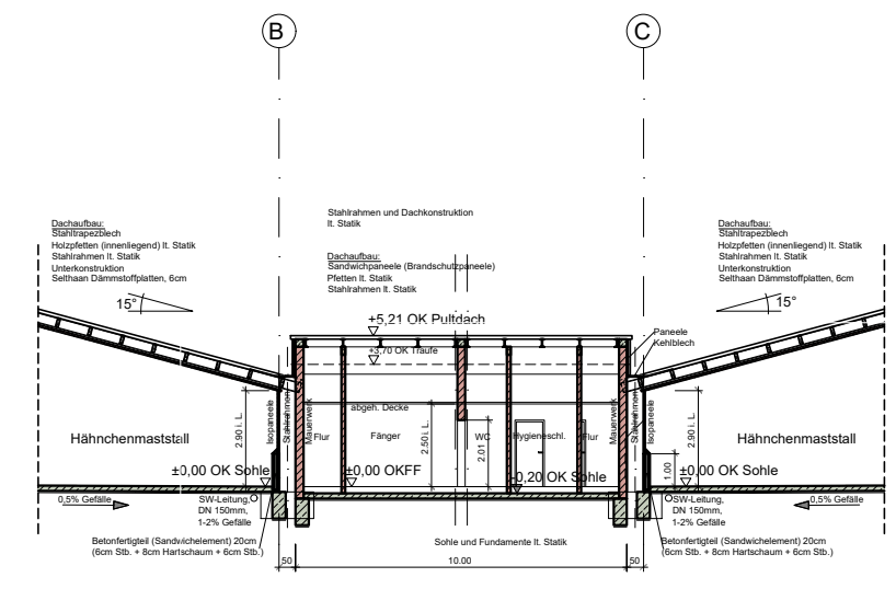
Schnitt E-E
