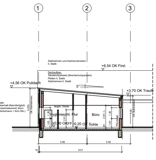
Schnitt D-D
