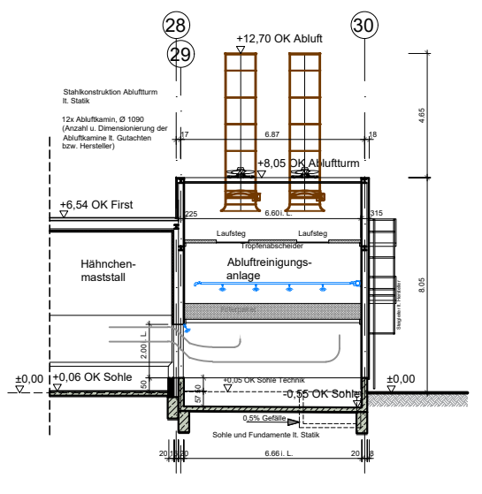
Schnitt C-C
